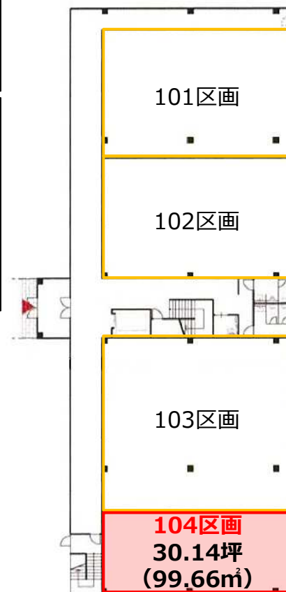
1F 平面図
